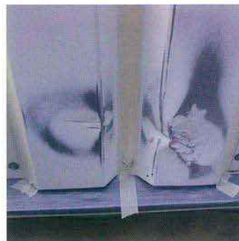
Typisches Schadensbild: Fenster-Festelement (RAL 7016) vor und nach der Reparatur.
